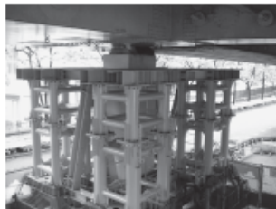
鋼製ベント・サンドル材
