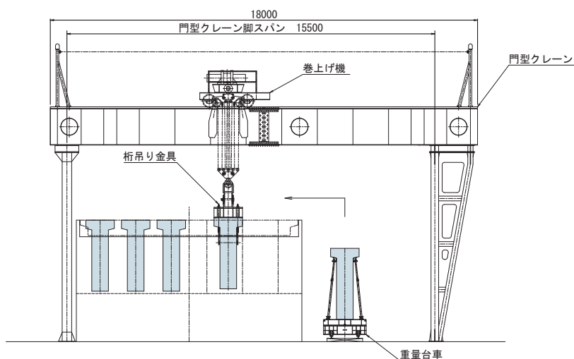
門型クレーン断面図
