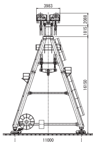
門型クレーン側面図
