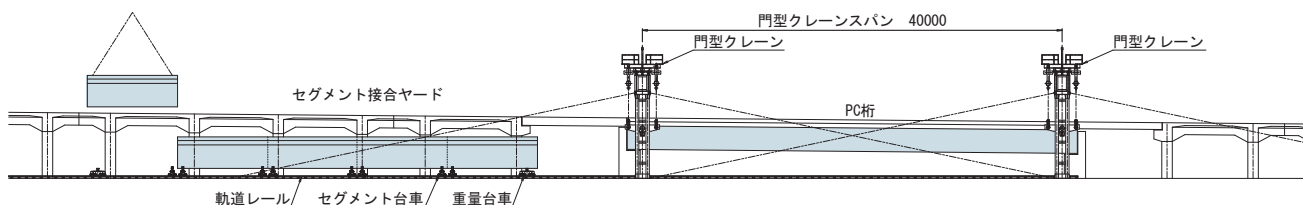
側面図
