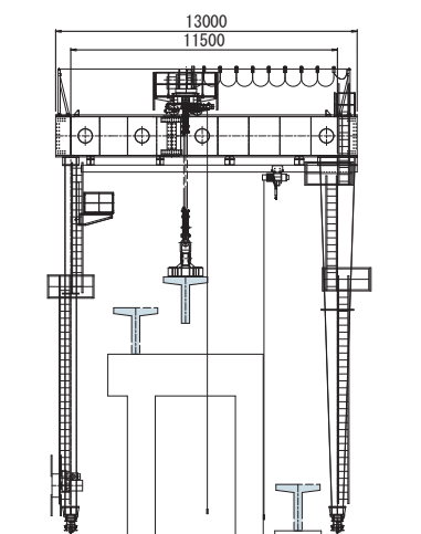
門型クレーン断面図
