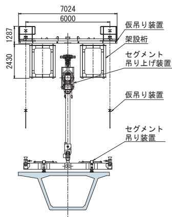
セグメント吊り金具断面図
