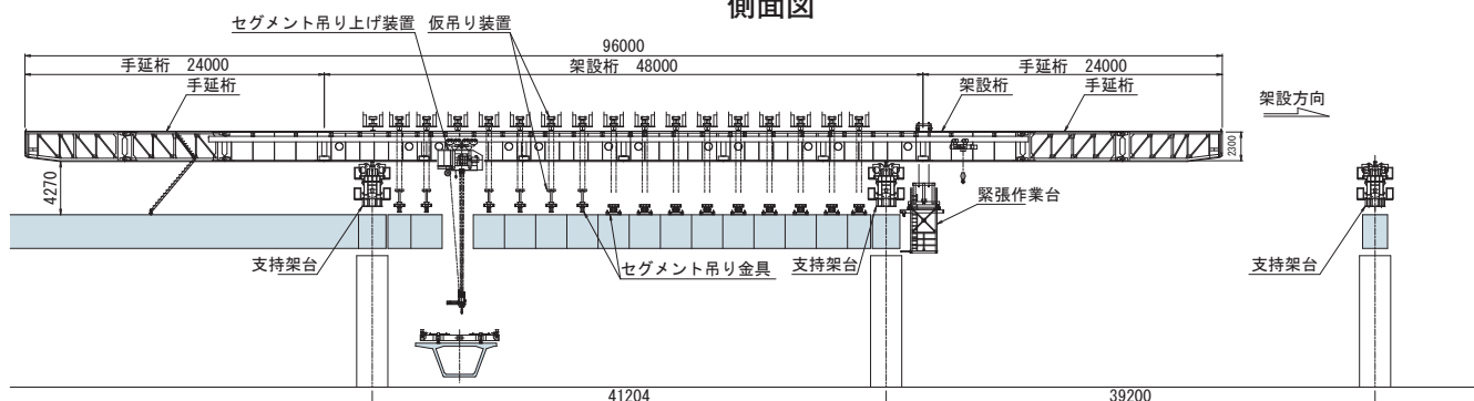
側面図
