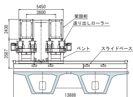
支持架台断面図
