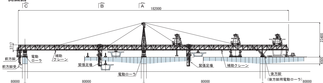
側面図
