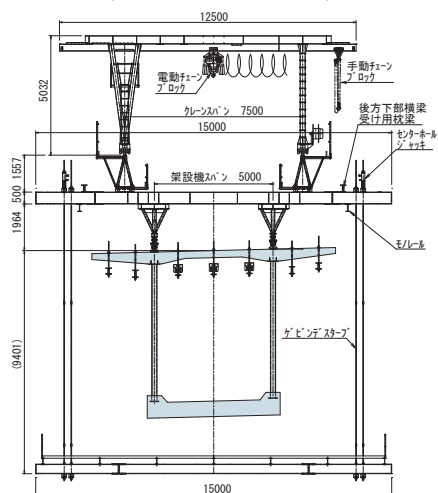
A断面 (後方上部横梁断面)
