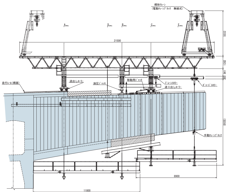
A断面 (後方上部横梁断面)
