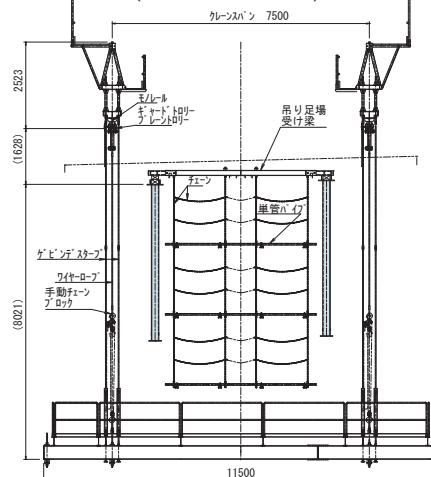
E断面 (スライダ足場断面)
