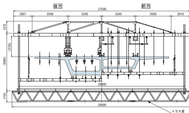
3主構
