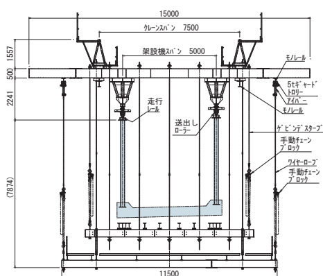
C断面 (前方上部横梁断面)
