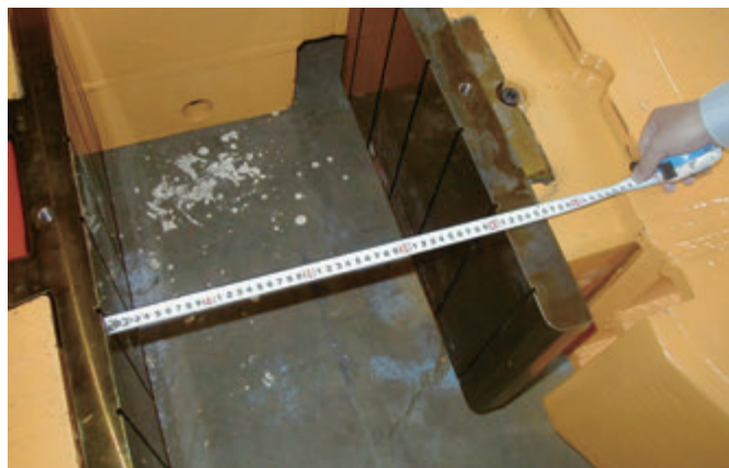
PC矢板用チャック 爪部
