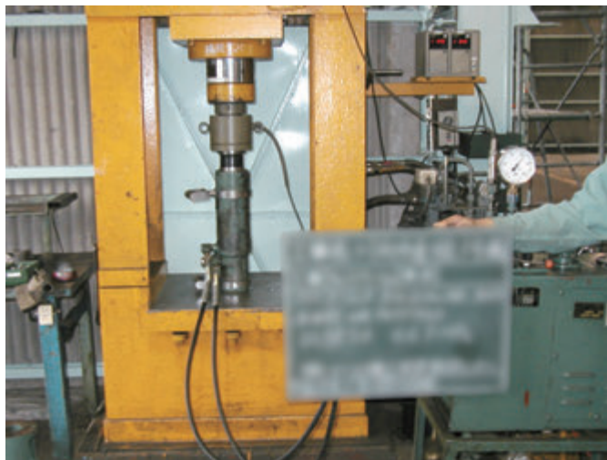
ストランド緊張ジャッキのキャリブレーション
