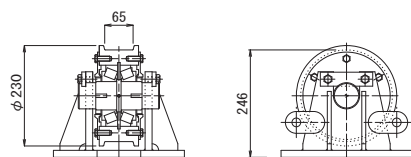
20 t シングル
