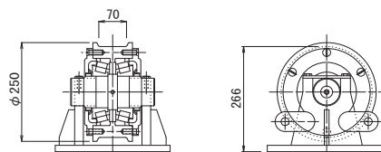
30 t シングル
