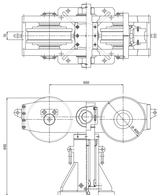
100 t ジャッキ付き・安全ナット付き
