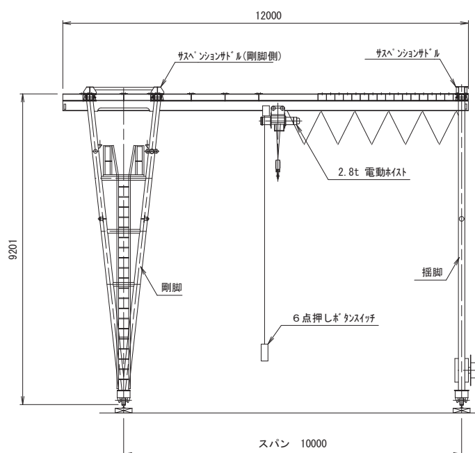
正面図
