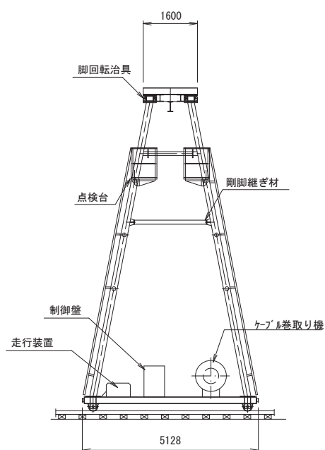
側面図
