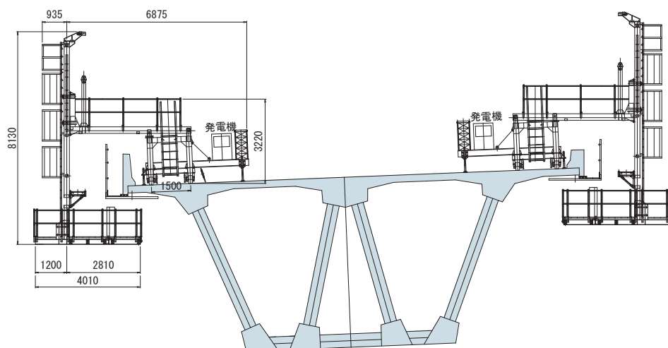
断面図
