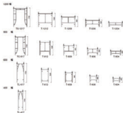
建枠一覧表
