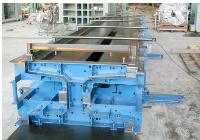
鋼製型枠(H型PC杭)
