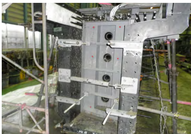
鋼製型枠(セグメント桁)
